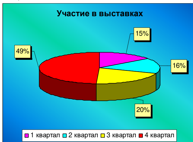
Рисунок 4. Образец круговой диаграммы
